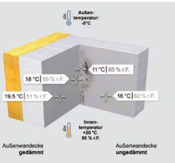
Oberflächentemperaturen [°C] und Luftfeuchte [%] der Innenseite einer Außenwand bei gedämmter und ungedämmter Außenwand
